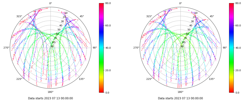
Skyplot for station VIGO. Parameter M1C Data file VIGO00ESP_R_2023194.xtr Skyplot for station VIGO. Parameter M2C Data file VIGO00ESP_R_2023194.xtr
