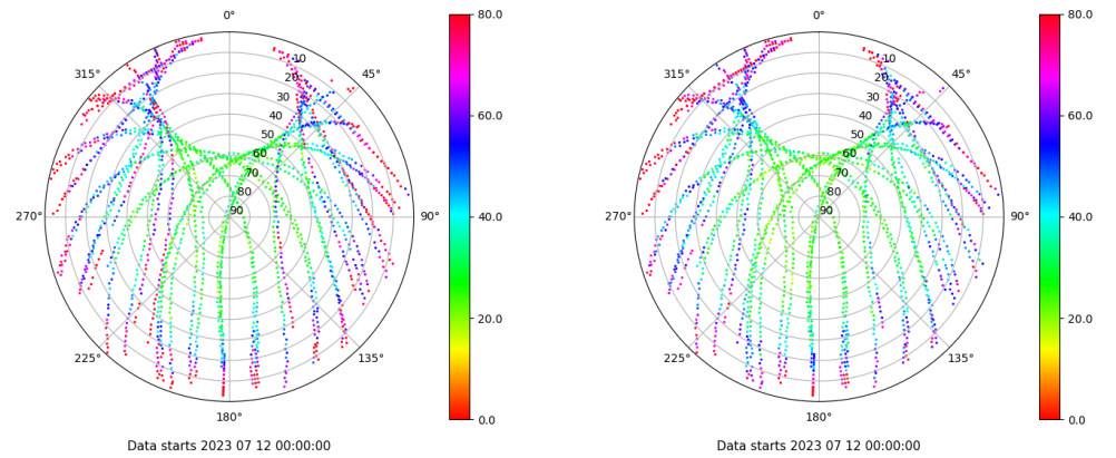
Skyplot for station VIGO. Parameter M1C Data file VIGO00ESP_R_2023193.xtr Skyplot for station VIGO. Parameter M2C Data file VIGO00ESP_R_2023193.xtr
