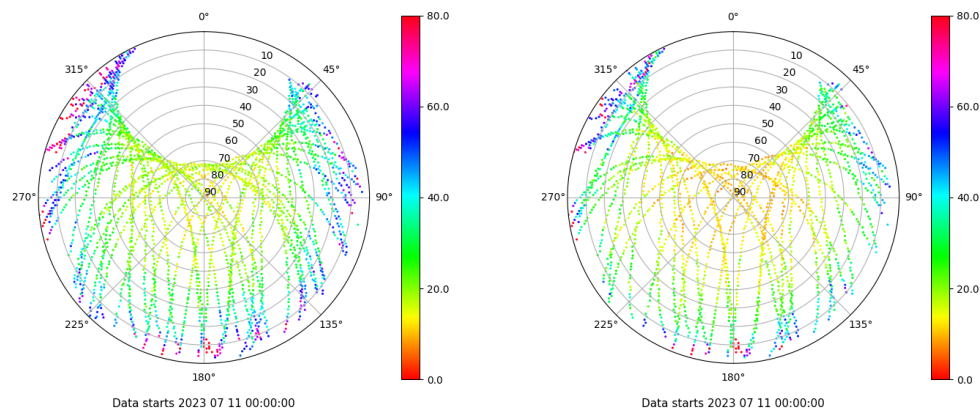
Skyplot for station VIGO. Parameter M1C Data file VIGO00ESP_R_2023192.xtr Skyplot for station VIGO. Parameter M2X Data file VIGO00ESP_R_2023192.xtr
