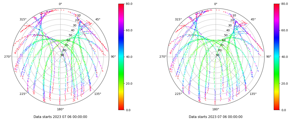
Skyplot for station VIGO. Parameter M1C Data file VIGO00ESP_R_2023187.xtr Skyplot for station VIGO. Parameter M2C Data file VIGO00ESP_R_2023187.xtr
