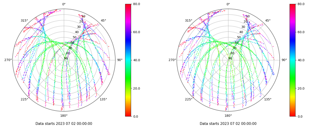
Skyplot for station VIGO. Parameter M1C Data file VIGO00ESP_R_2023183.xtr Skyplot for station VIGO. Parameter M2C Data file VIGO00ESP_R_2023183.xtr
