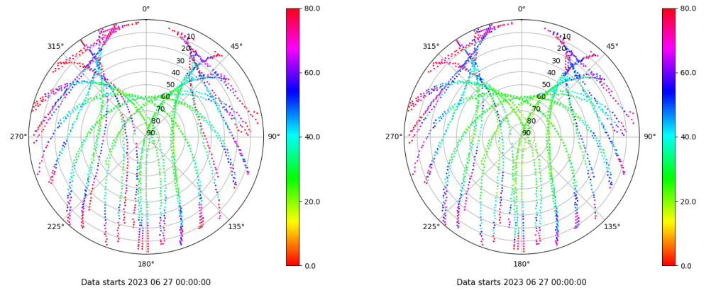
Skyplot for station VIGO. Parameter M1C Data file VIGO00ESP_R_2023178.xtr Skyplot for station VIGO. Parameter M2C Data file VIGO00ESP_R_2023178.xtr
