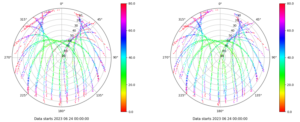
Skyplot for station VIGO. Parameter M1C Data file VIGO00ESP_R_2023175.xtr Skyplot for station VIGO. Parameter M2C Data file VIGO00ESP_R_2023175.xtr
