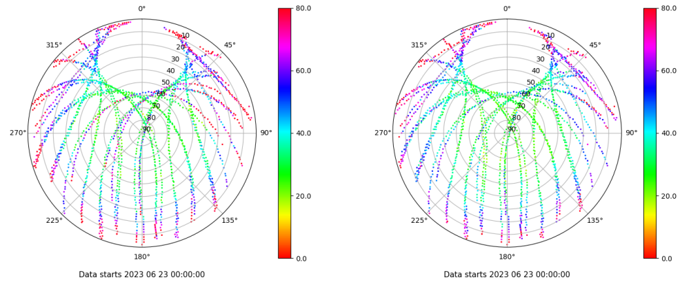
Skyplot for station VIGO. Parameter M1C Data file VIGO00ESP_R_2023174.xtr Skyplot for station VIGO. Parameter M2C Data file VIGO00ESP_R_2023174.xtr
