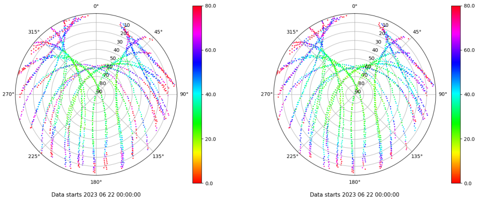
Skyplot for station VIGO. Parameter M1C Data file VIGO00ESP_R_2023173.xtr Skyplot for station VIGO. Parameter M2C Data file VIGO00ESP_R_2023173.xtr
