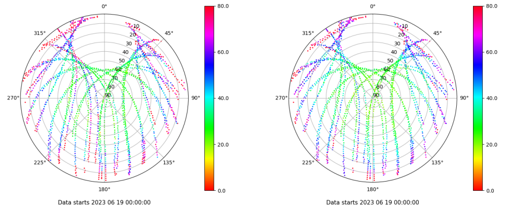
Skyplot for station VIGO. Parameter M1C Data file VIGO00ESP_R_2023170.xtr Skyplot for station VIGO. Parameter M2C Data file VIGO00ESP_R_2023170.xtr
