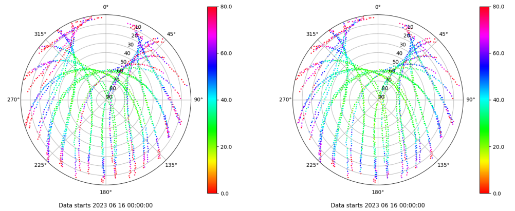
Skyplot for station VIGO. Parameter M1C Data file VIGO00ESP_R_2023167.xtr Skyplot for station VIGO. Parameter M2C Data file VIGO00ESP_R_2023167.xtr
