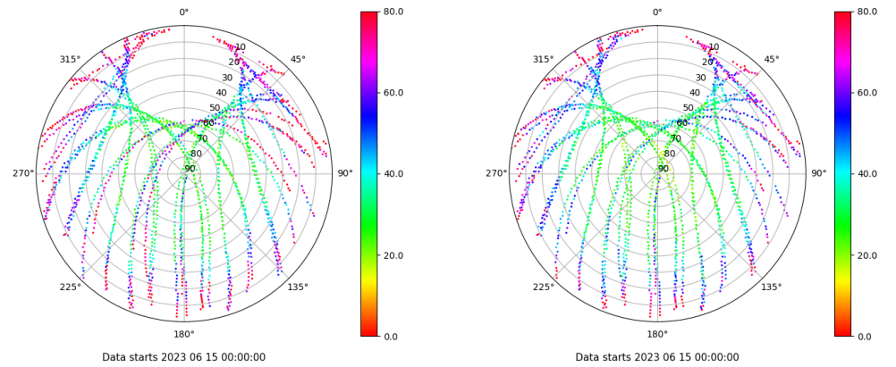
Skyplot for station VIGO. Parameter M1C Data file VIGO00ESP_R_2023166.xtr Skyplot for station VIGO. Parameter M2C Data file VIGO00ESP_R_2023166.xtr
