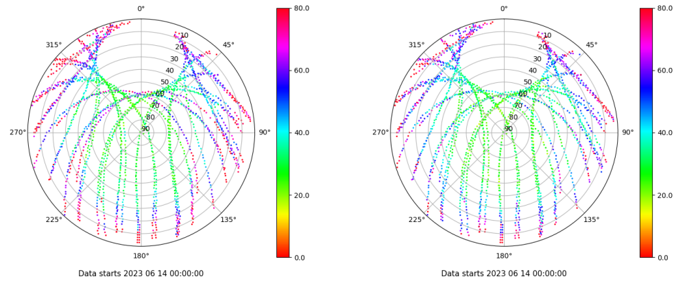
Skyplot for station VIGO. Parameter M1C Data file VIGO00ESP_R_2023165.xtr Skyplot for station VIGO. Parameter M2C Data file VIGO00ESP_R_2023165.xtr
