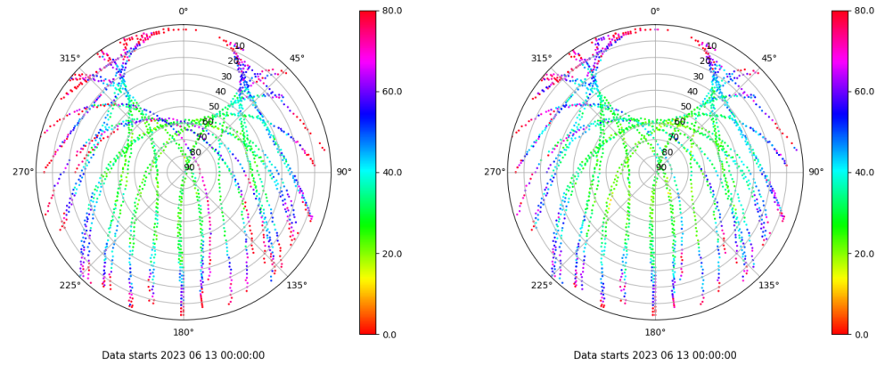
Skyplot for station VIGO. Parameter M1C Data file VIGO00ESP_R_2023164.xtr Skyplot for station VIGO. Parameter M2C Data file VIGO00ESP_R_2023164.xtr
