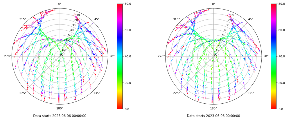
Skyplot for station VIGO. Parameter M1C Data file VIGO00ESP_R_2023157.xtr Skyplot for station VIGO. Parameter M2C Data file VIGO00ESP_R_2023157.xtr
