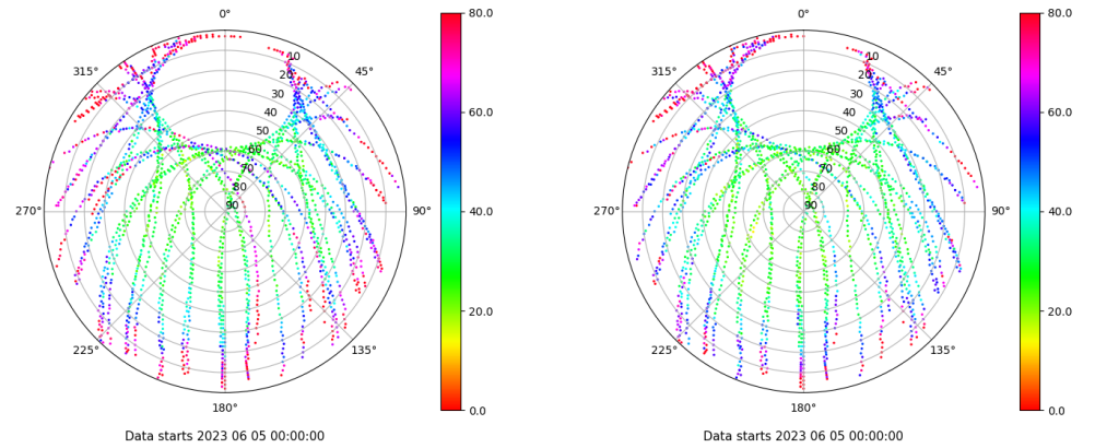
Skyplot for station VIGO. Parameter M1C Data file VIGO00ESP_R_2023156.xtr Skyplot for station VIGO. Parameter M2C Data file VIGO00ESP_R_2023156.xtr
