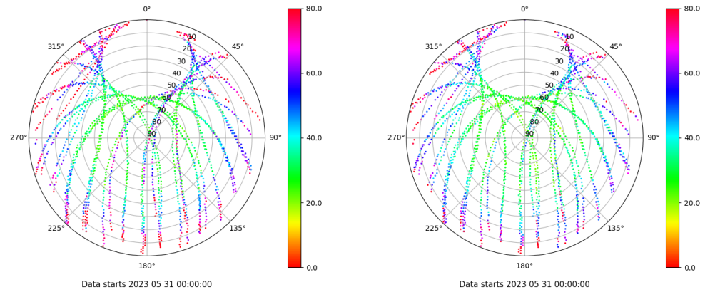
Skyplot for station VIGO. Parameter M1C Data file VIGO00ESP_R_2023151.xtr Skyplot for station VIGO. Parameter M2C Data file VIGO00ESP_R_2023151.xtr
