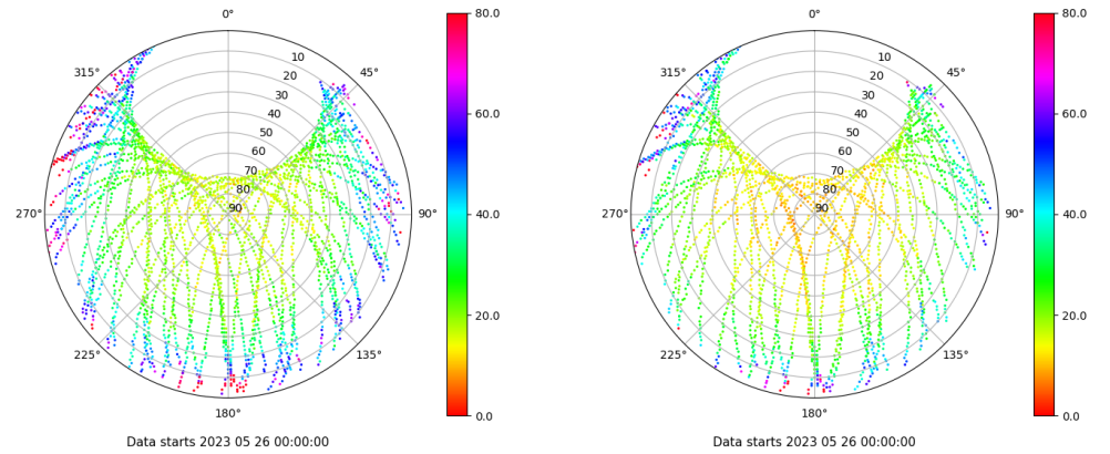
Skyplot for station VIGO. Parameter M1C Data file VIGO00ESP_R_2023146.xtr Skyplot for station VIGO. Parameter M2X Data file VIGO00ESP_R_2023146.xtr
