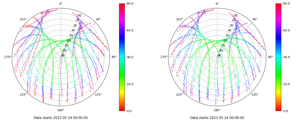
Skyplot for station VIGO. Parameter M1C Data file VIGO00ESP_R_2023144.xtr Skyplot for station VIGO. Parameter M2C Data file VIGO00ESP_R_2023144.xtr
