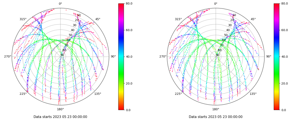
Skyplot for station VIGO. Parameter M1C Data file VIGO00ESP_R_2023143.xtr Skyplot for station VIGO. Parameter M2C Data file VIGO00ESP_R_2023143.xtr
