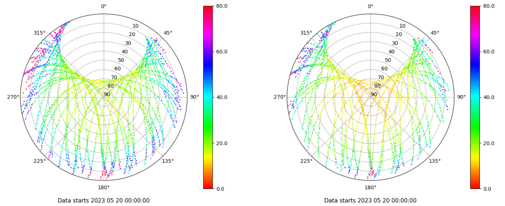
Skyplot for station VIGO. Parameter M1C Data file VIGO00ESP_R_2023140.xtr Skyplot for station VIGO. Parameter M2X Data file VIGO00ESP_R_2023140.xtr
