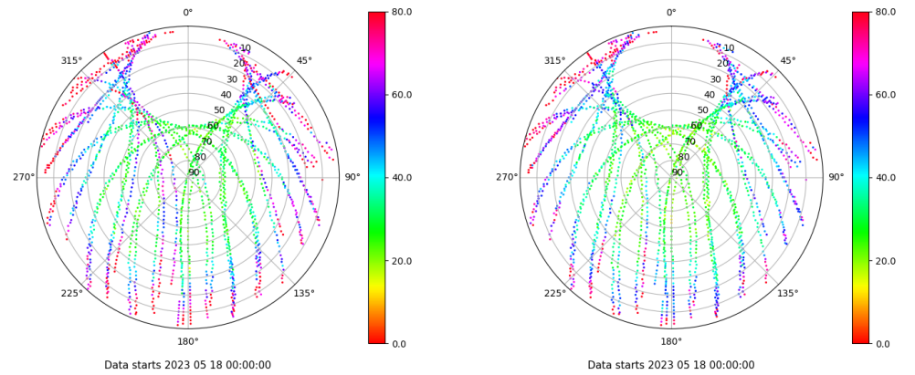
Skyplot for station VIGO. Parameter M1C Data file VIGO00ESP_R_2023138.xtr Skyplot for station VIGO. Parameter M2C Data file VIGO00ESP_R_2023138.xtr
