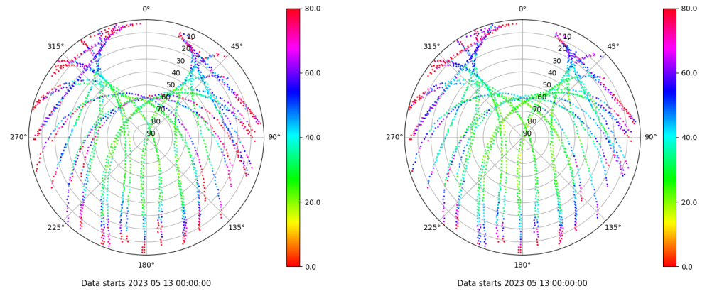
Skyplot for station VIGO. Parameter M1C Data file VIGO00ESP_R_2023133.xtr Skyplot for station VIGO. Parameter M2C Data file VIGO00ESP_R_2023133.xtr
