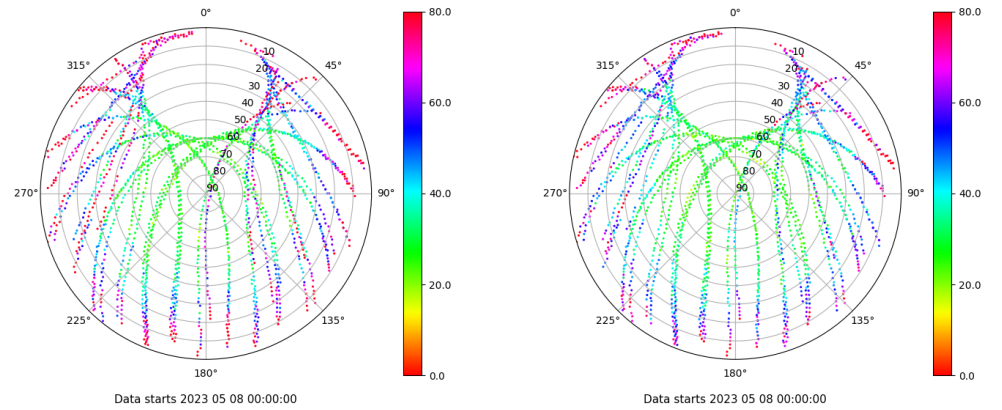
Skyplot for station VIGO. Parameter M1C Data file VIGO00ESP_R_2023128.xtr Skyplot for station VIGO. Parameter M2C Data file VIGO00ESP_R_2023128.xtr
