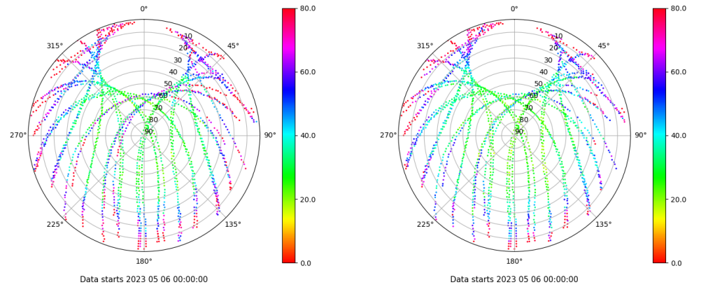
Skyplot for station VIGO. Parameter M1C Data file VIGO00ESP_R_2023126.xtr Skyplot for station VIGO. Parameter M2C Data file VIGO00ESP_R_2023126.xtr
