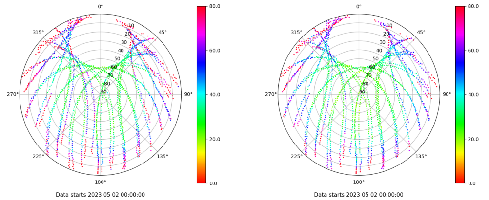
Skyplot for station VIGO. Parameter M1C Data file VIGO00ESP_R_2023122.xtr Skyplot for station VIGO. Parameter M2C Data file VIGO00ESP_R_2023122.xtr
