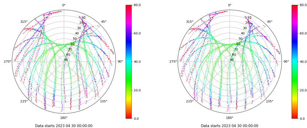
Skyplot for station VIGO. Parameter M1C Data file VIGO00ESP_R_2023120.xtr Skyplot for station VIGO. Parameter M2C Data file VIGO00ESP_R_2023120.xtr
