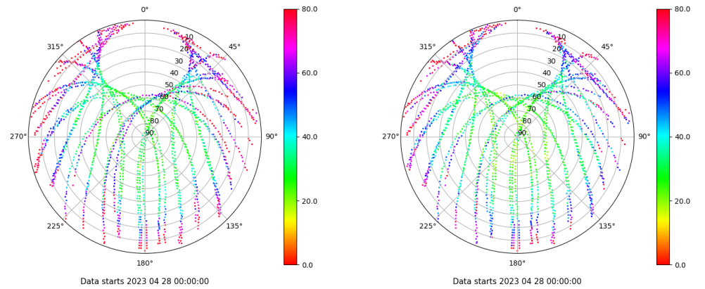
Skyplot for station VIGO. Parameter M1C Data file VIGO00ESP_R_2023118.xtr Skyplot for station VIGO. Parameter M2C Data file VIGO00ESP_R_2023118.xtr
