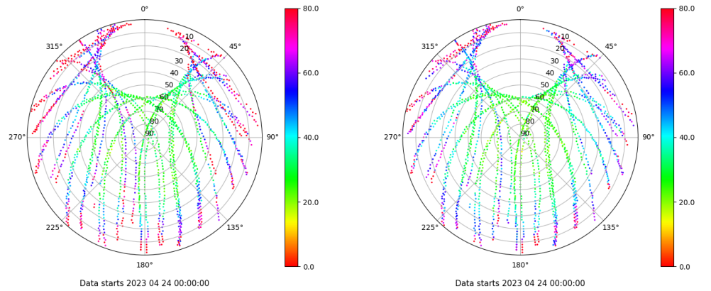
Skyplot for station VIGO. Parameter M1C Data file VIGO00ESP_R_2023114.xtr Skyplot for station VIGO. Parameter M2C Data file VIGO00ESP_R_2023114.xtr
