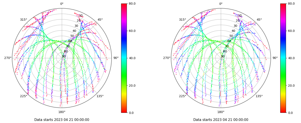
Skyplot for station VIGO. Parameter M1C Data file VIGO00ESP_R_2023111.xtr Skyplot for station VIGO. Parameter M2C Data file VIGO00ESP_R_2023111.xtr
