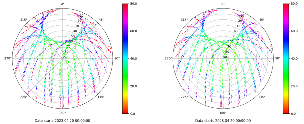
Skyplot for station VIGO. Parameter M1C Data file VIGO00ESP_R_2023110.xtr Skyplot for station VIGO. Parameter M2C Data file VIGO00ESP_R_2023110.xtr
