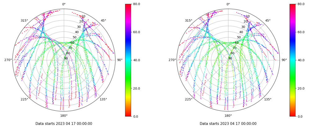
Skyplot for station VIGO. Parameter M1C Data file VIGO00ESP_R_2023107.xtr Skyplot for station VIGO. Parameter M2C Data file VIGO00ESP_R_2023107.xtr
