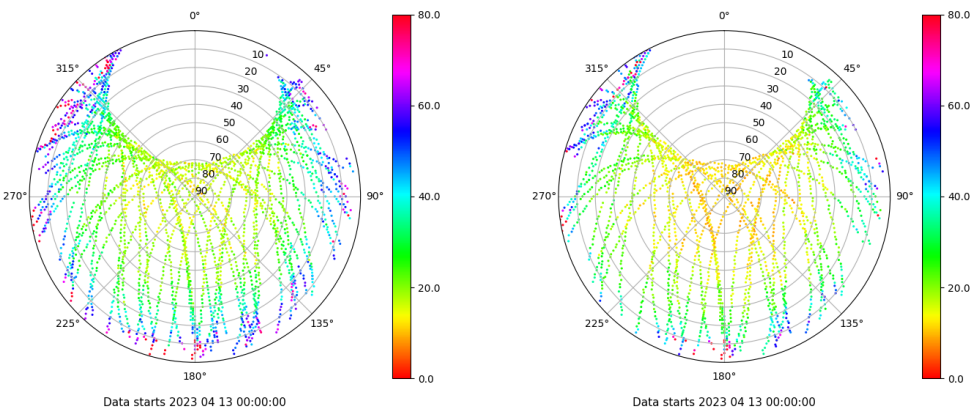
Skyplot for station VIGO. Parameter M1C Data file VIGO00ESP_R_2023103.xtr Skyplot for station VIGO. Parameter M2X Data file VIGO00ESP_R_2023103.xtr
