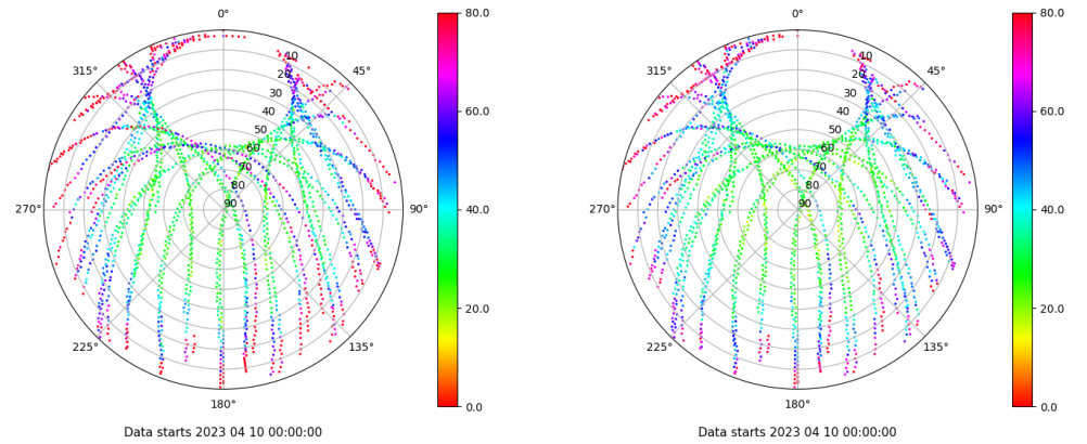
Skyplot for station VIGO. Parameter M1C Data file VIGO00ESP_R_2023100.xtr Skyplot for station VIGO. Parameter M2C Data file VIGO00ESP_R_2023100.xtr
