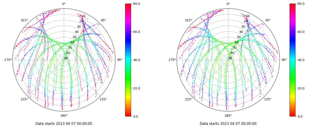
Skyplot for station VIGO. Parameter M1C Data file VIGO00ESP_R_2023097.xtr Skyplot for station VIGO. Parameter M2C Data file VIGO00ESP_R_2023097.xtr
