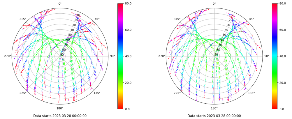
Skyplot for station VIGO. Parameter M1C Data file VIGO00ESP_R_2023087.xtr Skyplot for station VIGO. Parameter M2C Data file VIGO00ESP_R_2023087.xtr
