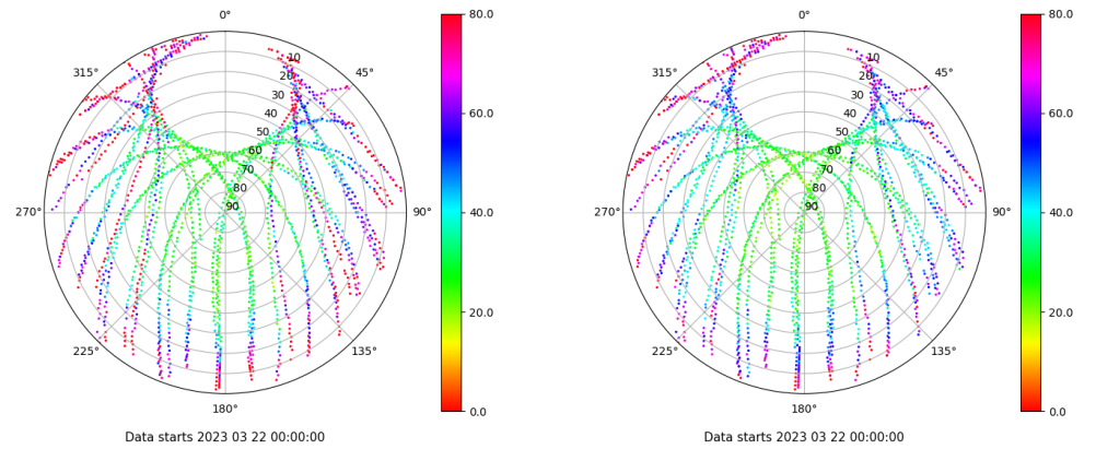
Skyplot for station VIGO. Parameter M1C Data file VIGO00ESP_R_2023081.xtr Skyplot for station VIGO. Parameter M2C Data file VIGO00ESP_R_2023081.xtr
