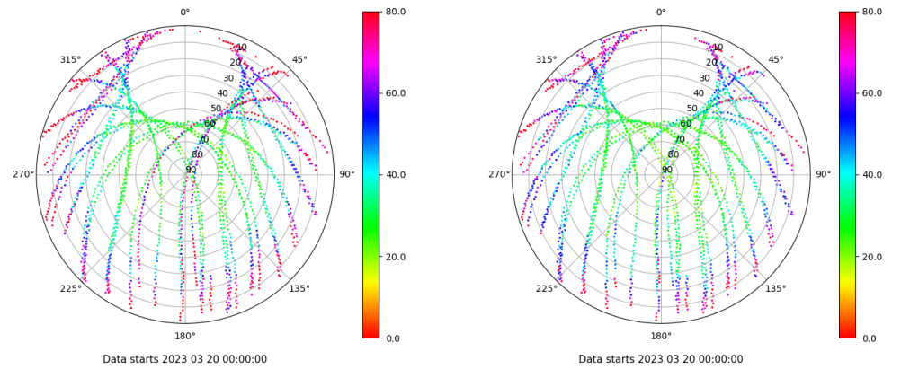
Skyplot for station VIGO. Parameter M1C Data file VIGO00ESP_R_2023079.xtr Skyplot for station VIGO. Parameter M2C Data file VIGO00ESP_R_2023079.xtr
