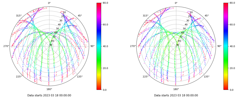
Skyplot for station VIGO. Parameter M1C Data file VIGO00ESP_R_2023077.xtr Skyplot for station VIGO. Parameter M2C Data file VIGO00ESP_R_2023077.xtr
