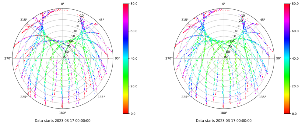
Skyplot for station VIGO. Parameter M1C Data file VIGO00ESP_R_2023076.xtr Skyplot for station VIGO. Parameter M2C Data file VIGO00ESP_R_2023076.xtr
