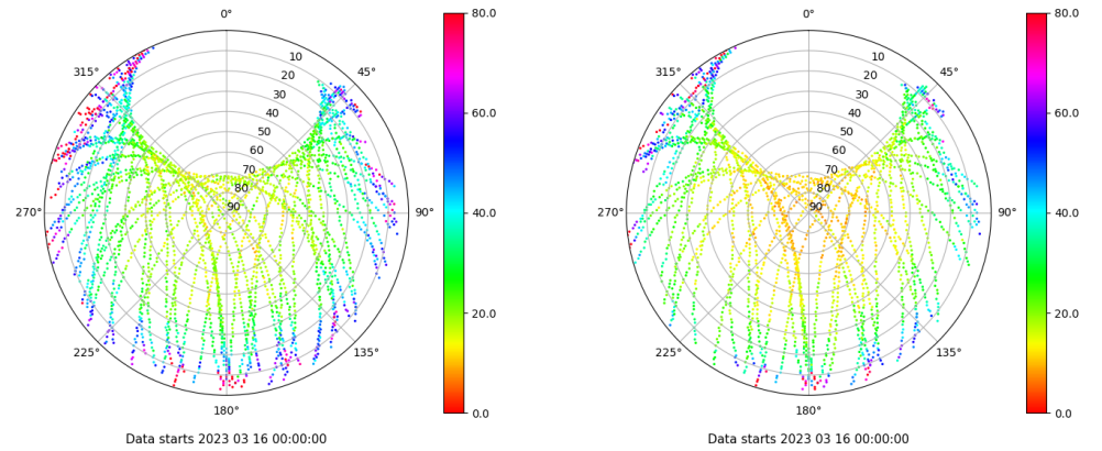
Skyplot for station VIGO. Parameter M1C Data file VIGO00ESP_R_2023075.xtr Skyplot for station VIGO. Parameter M2X Data file VIGO00ESP_R_2023075.xtr
