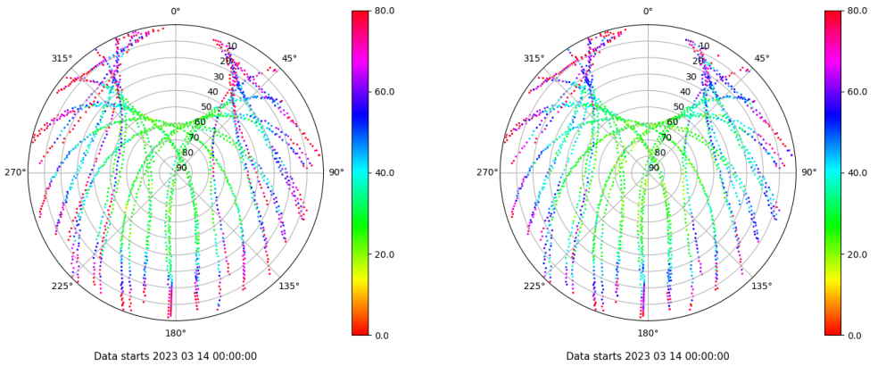
Skyplot for station VIGO. Parameter M1C Data file VIGO00ESP_R_2023073.xtr Skyplot for station VIGO. Parameter M2C Data file VIGO00ESP_R_2023073.xtr
