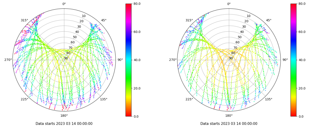
Skyplot for station VIGO. Parameter M1C Data file VIGO00ESP_R_2023073.xtr Skyplot for station VIGO. Parameter M2X Data file VIGO00ESP_R_2023073.xtr
