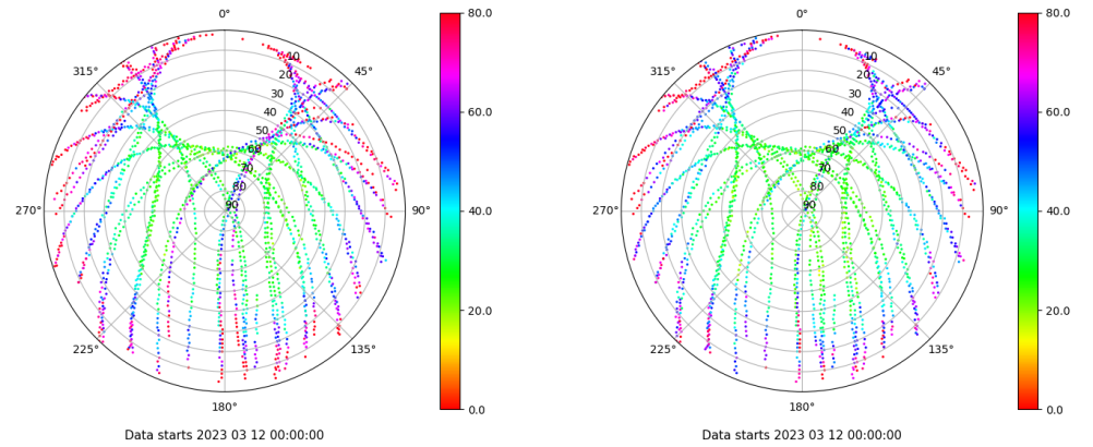
Skyplot for station VIGO. Parameter M1C Data file VIGO00ESP_R_2023071.xtr Skyplot for station VIGO. Parameter M2C Data file VIGO00ESP_R_2023071.xtr
