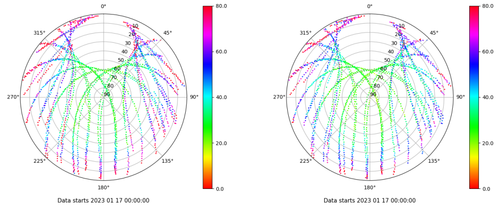
Skyplot for station VIGO. Parameter M1C Data file VIGO00ESP_R_2023017.xtr Skyplot for station VIGO. Parameter M2C Data file VIGO00ESP_R_2023017.xtr
