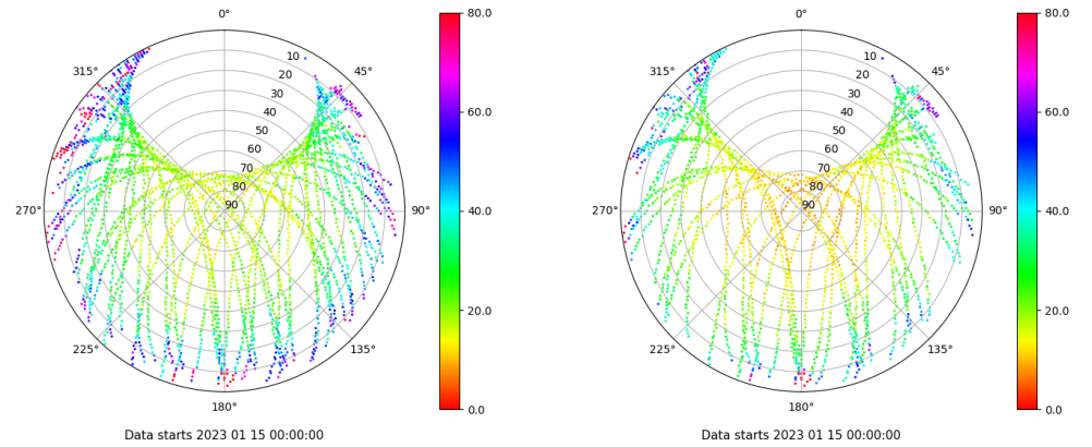
Skyplot for station VIGO. Parameter M1C Data file VIGO00ESP_R_2023015.xtr Skyplot for station VIGO. Parameter M2X Data file VIGO00ESP_R_2023015.xtr
