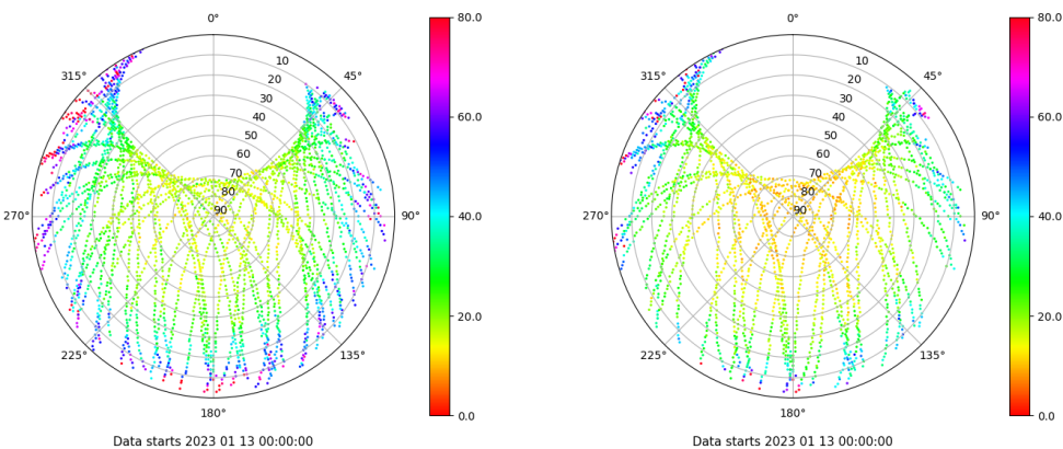
Skyplot for station VIGO. Parameter M1C Data file VIGO00ESP_R_2023013.xtr Skyplot for station VIGO. Parameter M2X Data file VIGO00ESP_R_2023013.xtr
