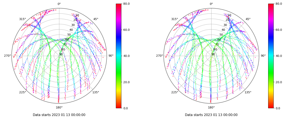
Skyplot for station VIGO. Parameter M1C Data file VIGO00ESP_R_2023013.xtr Skyplot for station VIGO. Parameter M2C Data file VIGO00ESP_R_2023013.xtr
