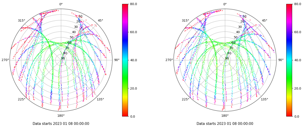
Skyplot for station VIGO. Parameter M1C Data file VIGO00ESP_R_2023008.xtr Skyplot for station VIGO. Parameter M2C Data file VIGO00ESP_R_2023008.xtr
