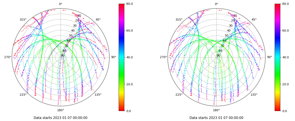
Skyplot for station VIGO. Parameter M1C Data file VIGO00ESP_R_2023007.xtr Skyplot for station VIGO. Parameter M2C Data file VIGO00ESP_R_2023007.xtr
