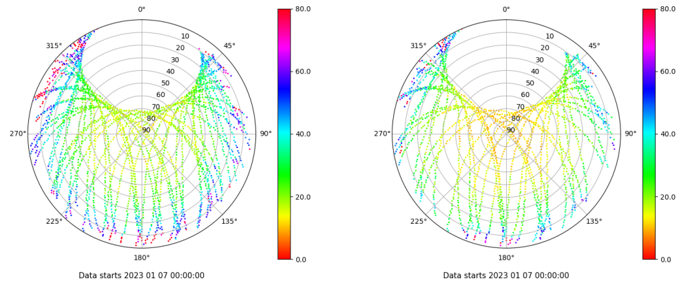
Skyplot for station VIGO. Parameter M1C Data file VIGO00ESP_R_2023007.xtr Skyplot for station VIGO. Parameter M2X Data file VIGO00ESP_R_2023007.xtr
