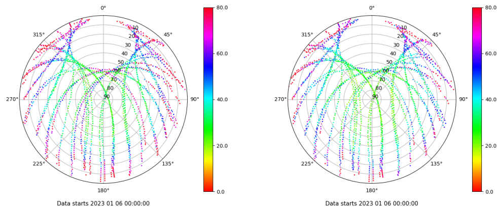
Skyplot for station VIGO. Parameter M1C Data file VIGO00ESP_R_2023006.xtr Skyplot for station VIGO. Parameter M2C Data file VIGO00ESP_R_2023006.xtr
