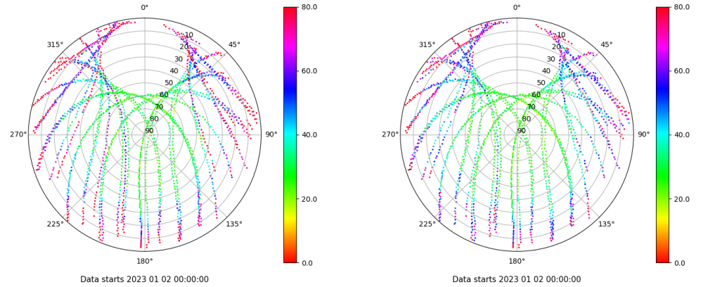
Skyplot for station VIGO. Parameter M1C Data file VIGO00ESP_R_2023002.xtr Skyplot for station VIGO. Parameter M2C Data file VIGO00ESP_R_2023002.xtr
